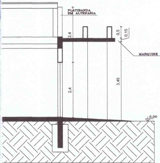
CORTE BB Escala 1/100
