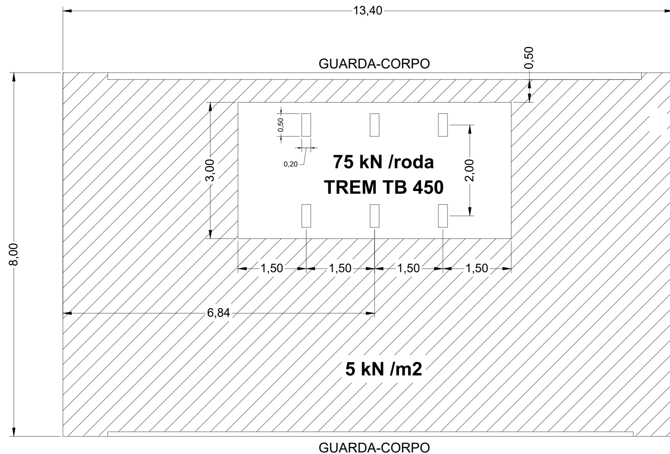
POSIÇÃO DO TREM TIPO TB 450
